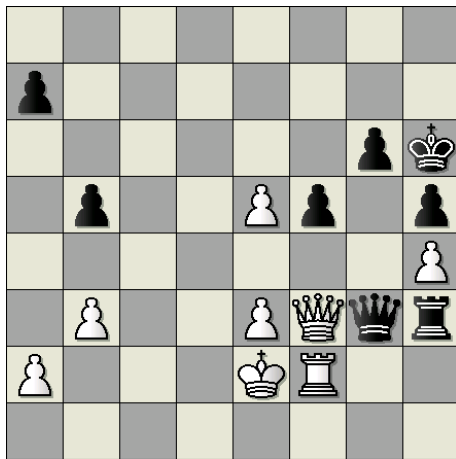
Analysediagram na 50. Df3
